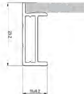
SEKCE-KRÁTKÁ STRANA
